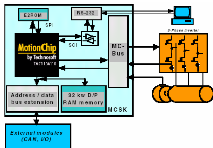
MotionChip 運動控制系統框圖
