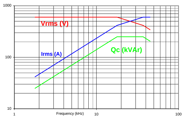
C200T 6.2μF - 600 Vrms - 600 Arms - 250 kVAr
