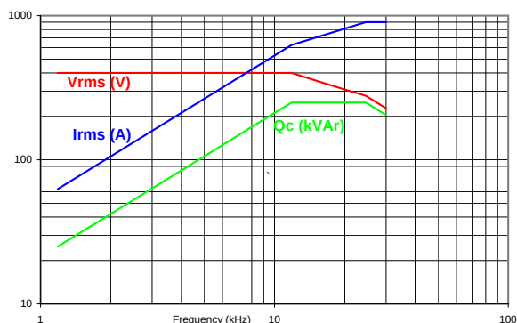
C200T 21μF - 400 Vrms - 900 Arms - 250 kVAr
