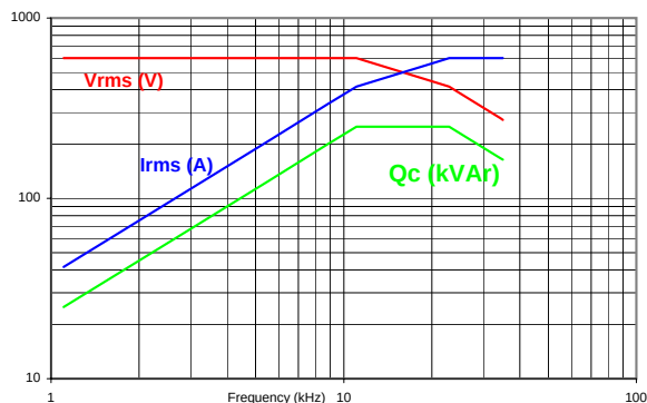
C200T 10μF - 600 Vrms - 600 Arms - 250 kVAr
