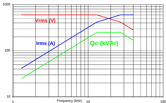
C200T 8.5μF - 600 Vrms - 600 Arms - 250 kVAr
