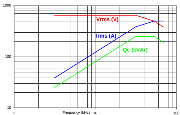
C200T 3μF - 650 Vrms - 500 Arms - 250 kVAr
