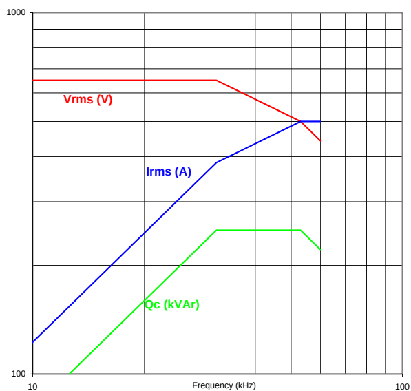
CSP300 3μF - 650 Vrms - 500 Arms - 250 kVAR
