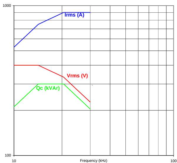
CSP300 21μF - 400 Vrms - 900 Arms - 300 kVAR
