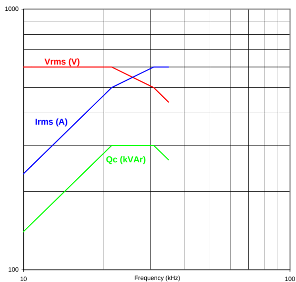
CSP300 6.2μF - 600 Vrms - 600 Arms - 300 kVAR
