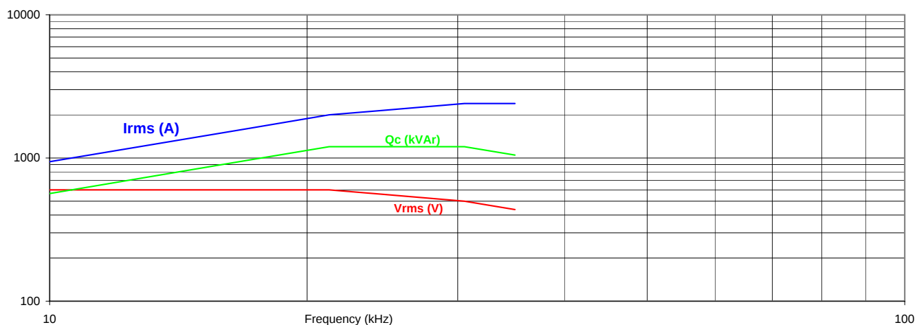
CSP1200 25µF - 600 Vrms - 2400 Arms - 1200 kVAr
