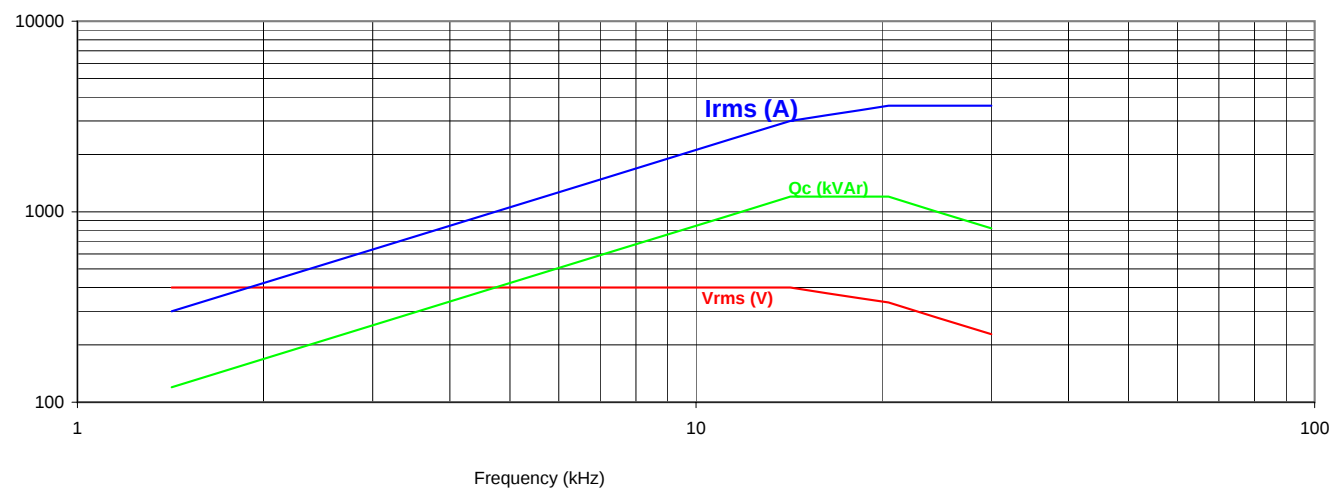
CSP1200 84µF - 400 Vrms - 3600 Arms - 1200 kVAr
