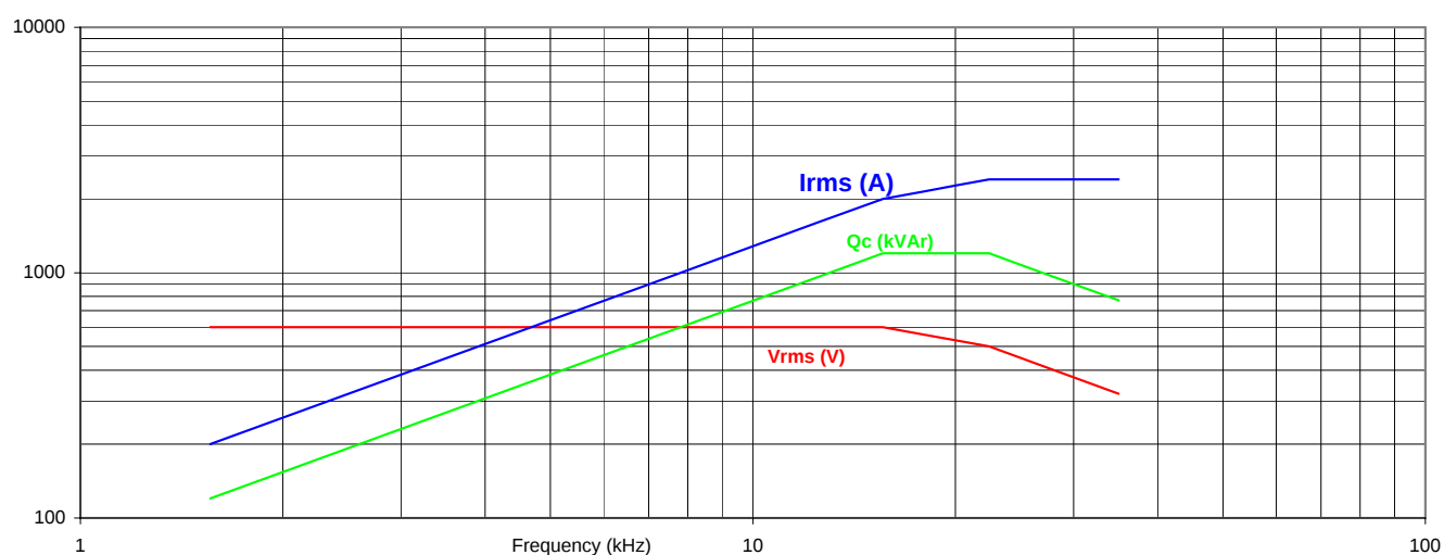
CSP1200 34µF - 600 Vrms - 2400 Arms - 1200 kVAr
